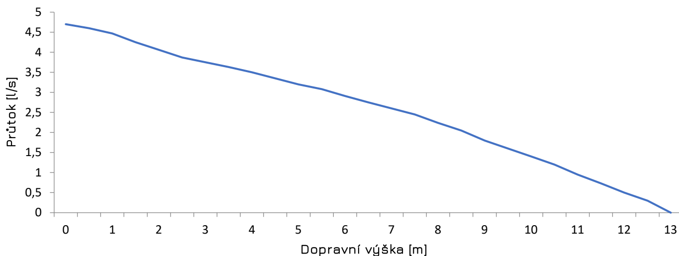
Q-H charakteristika pro čerpadlo PCH K2-T-280
